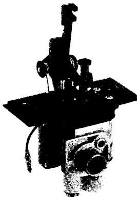
Schiebervergaser 81 ø 8
