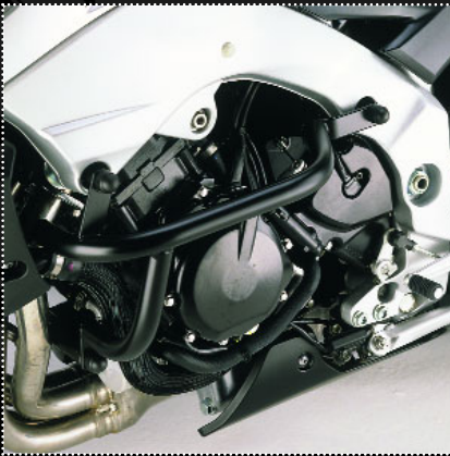
Schutzbügel „SE“ Protection Guard „SE“
